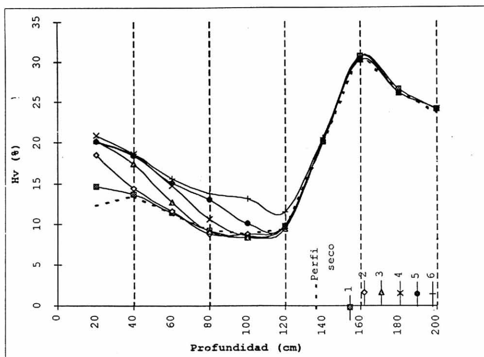
Figura 3. Perfiles hídricos levantados con sonda de neutrones durante el ensayo de infiltración en una de las posiciones del infiltrómetro de inundación por aspersion.
