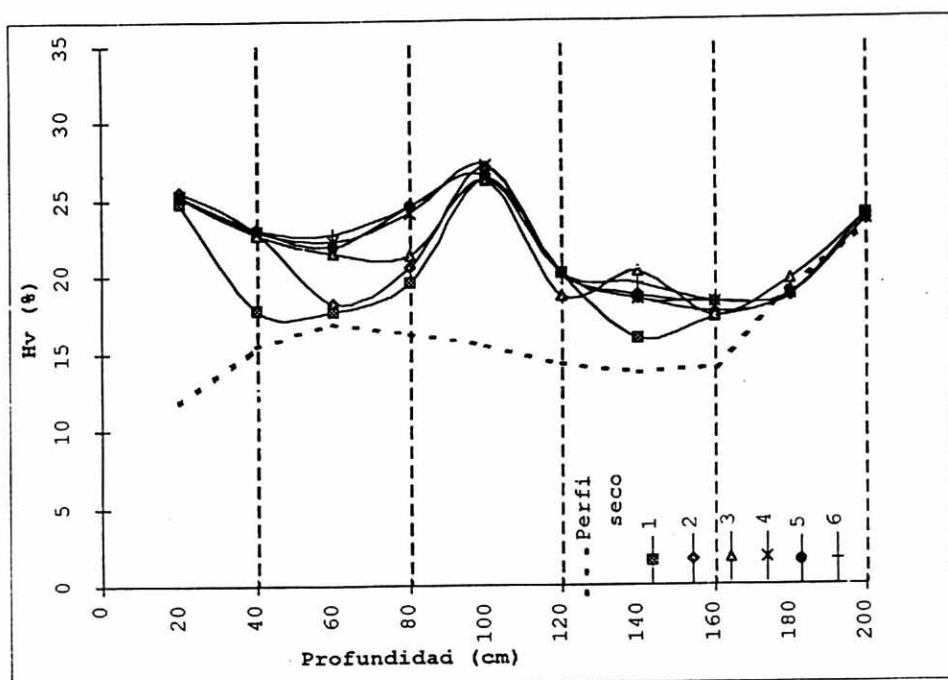
Figura 1. Perfiles hídricos levantados con sonda de neutrones durante el ensayo de infiltración en la posición 1 del doble anillo.
